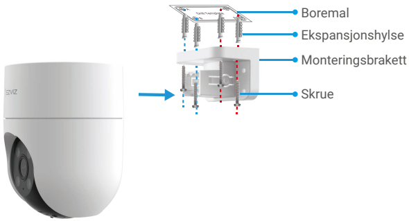
Fig. 1 Takmontering
